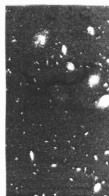
Andromedagalaxen har vuxit.
