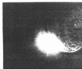
En bild från ögonblicket då kometen träffades.
